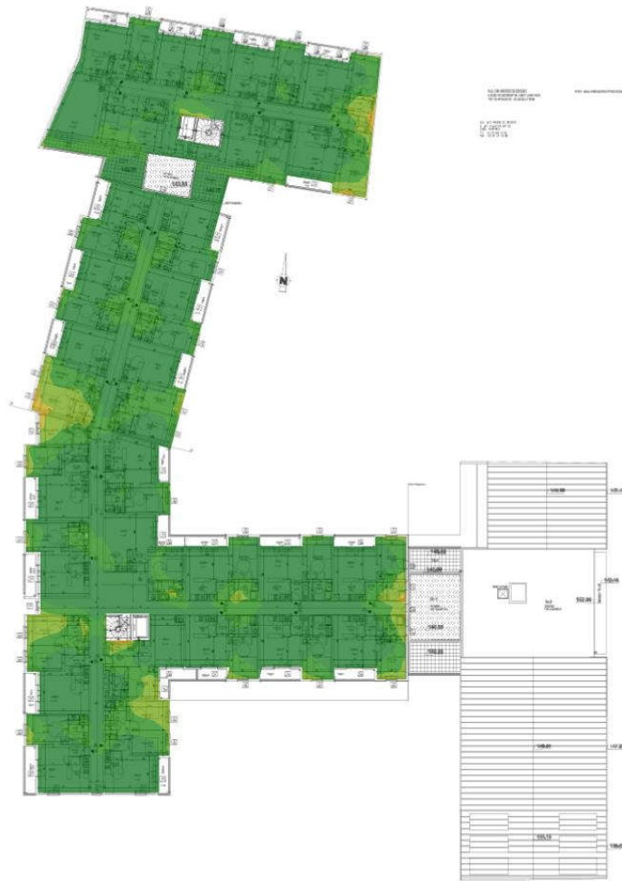
Figure 26 : CHARTRES-R+3 - Rapport signal sur bruit en 2.4Ghz
