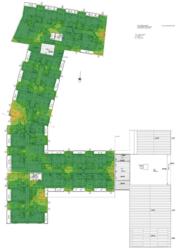
Figure 27 : CHARTRES-R+3 - Rapport signal sur bruit en 5GHZ
