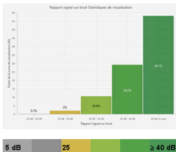
Figure 27 : CHARTRES-R+3 - Rapport signal sur bruit en 5GHZ
